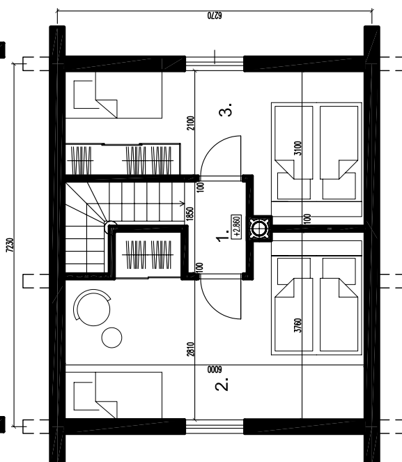
PÔDORYS PODKROVIA
